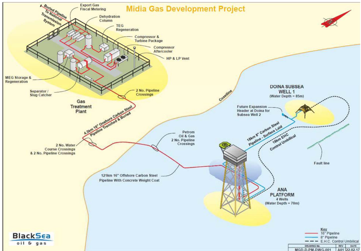
figura 1 Schema generală a Proiectului de Dezvoltare Gaze Naturale Midia
